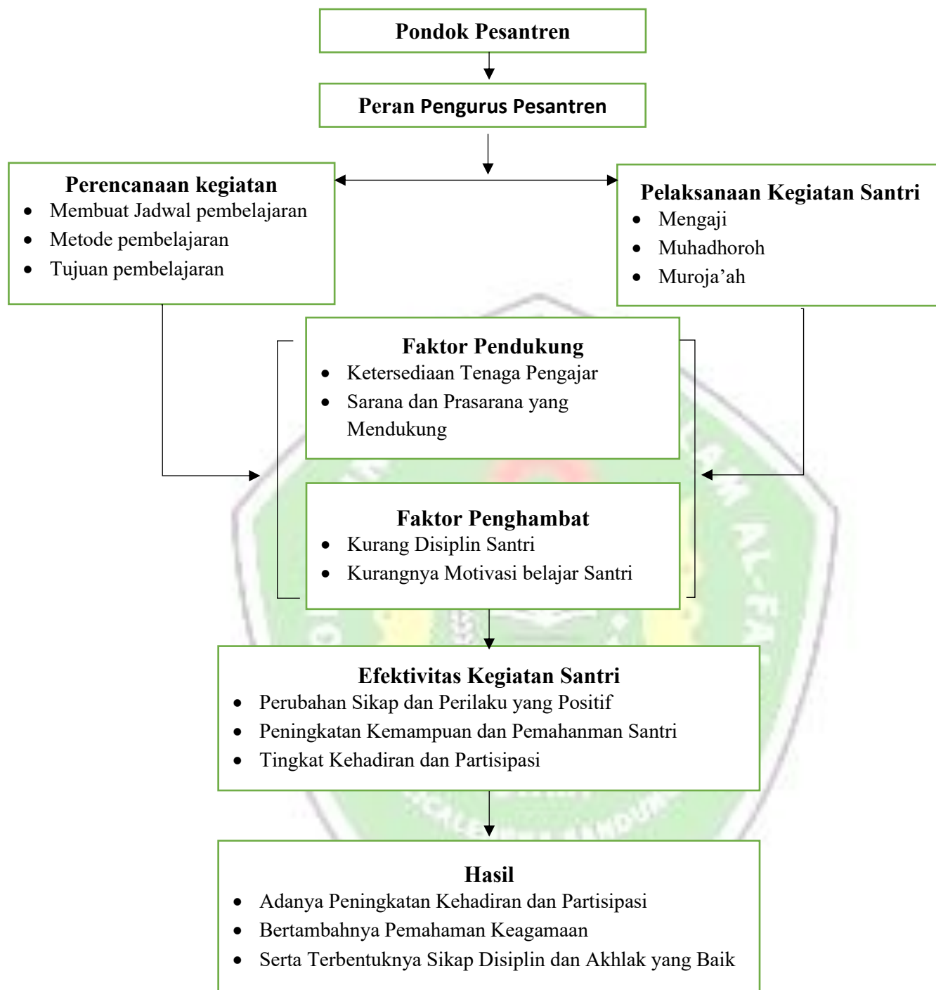
Gambar 1.1 Kerangka Berpikir
